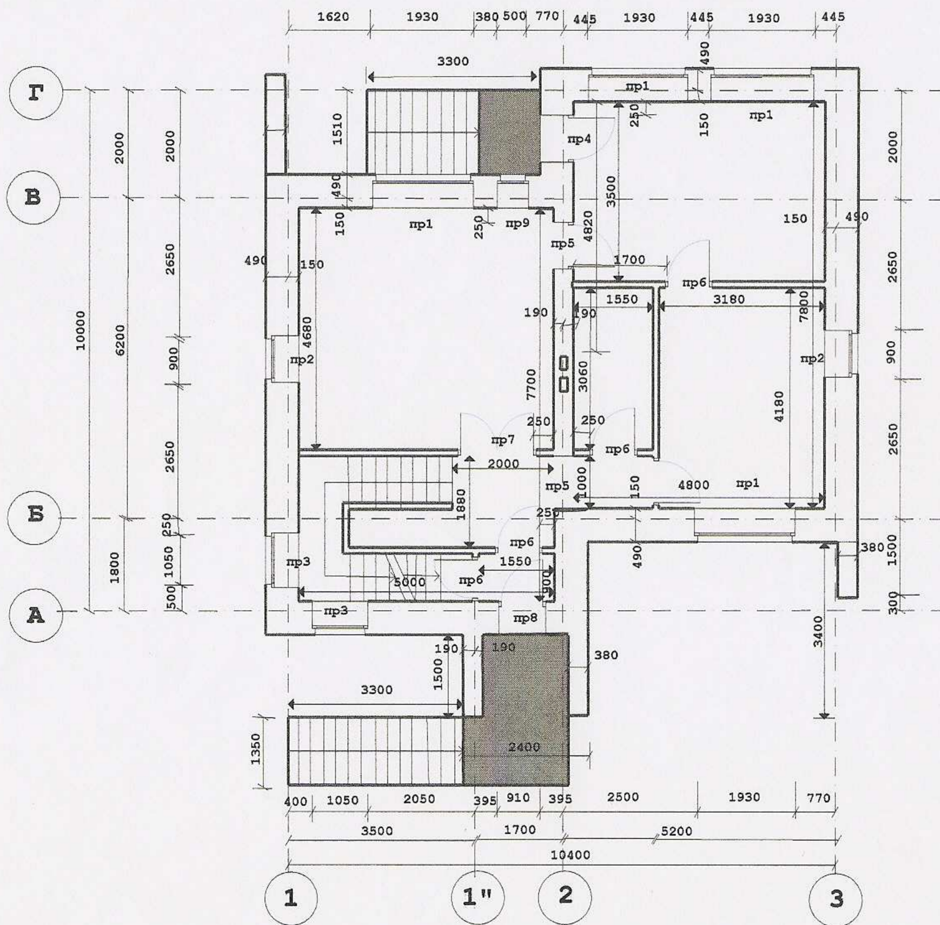
План 1 этажа
