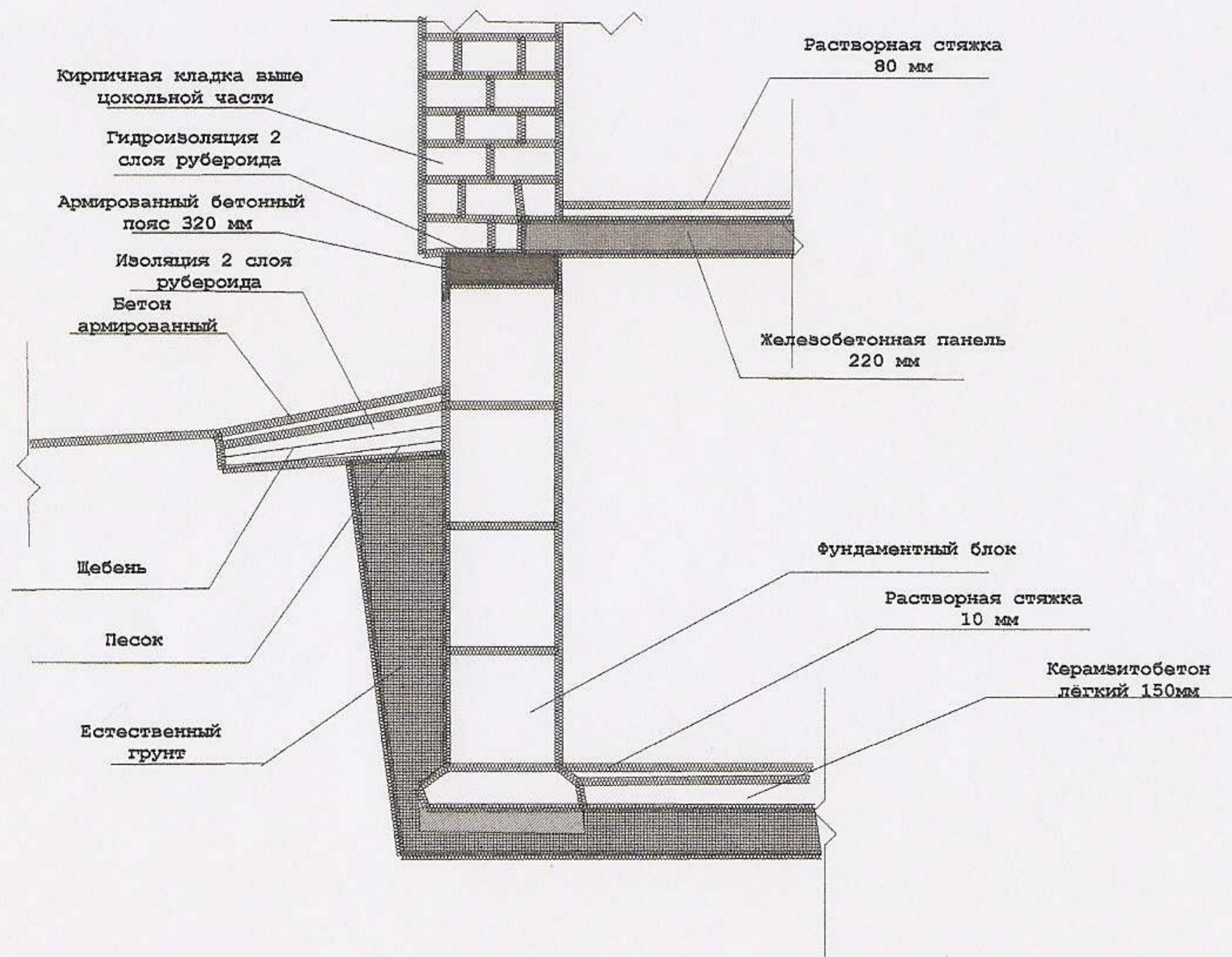
Разрез фундамента
