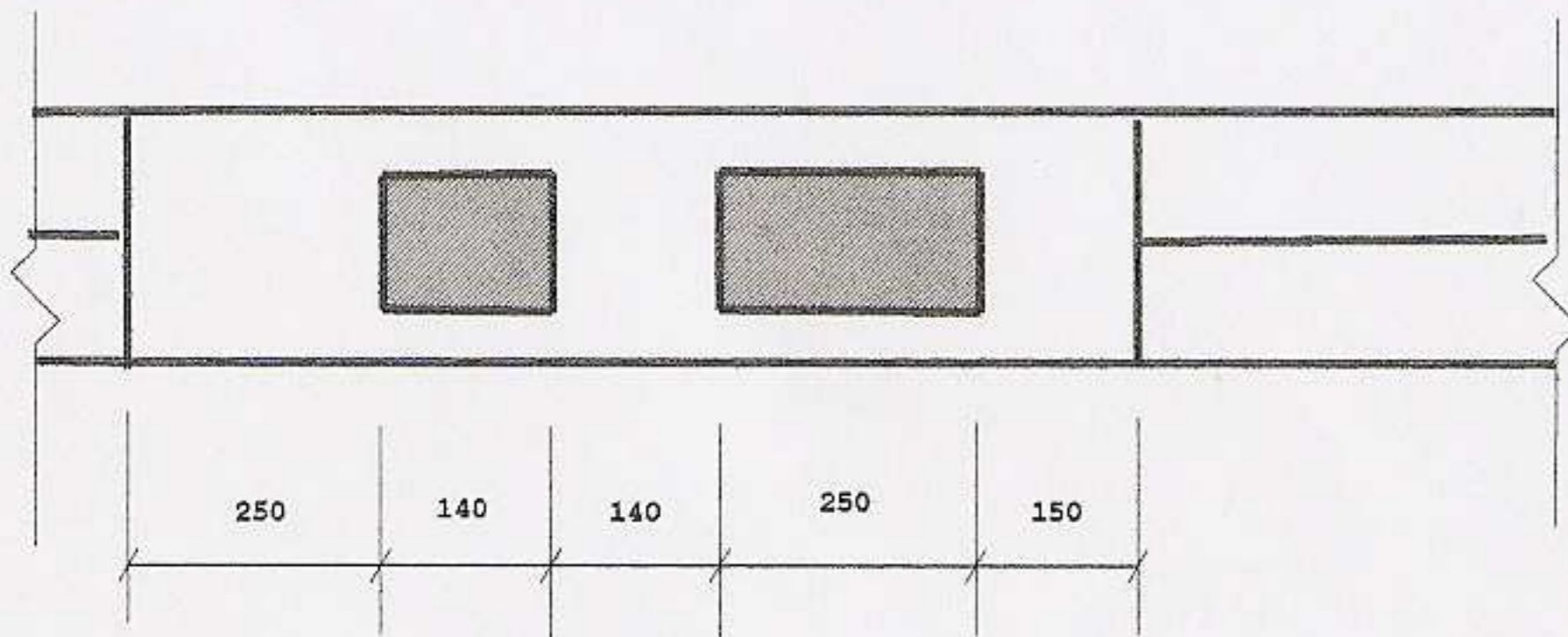
План вентиляц. канала и приёмн. трубы
