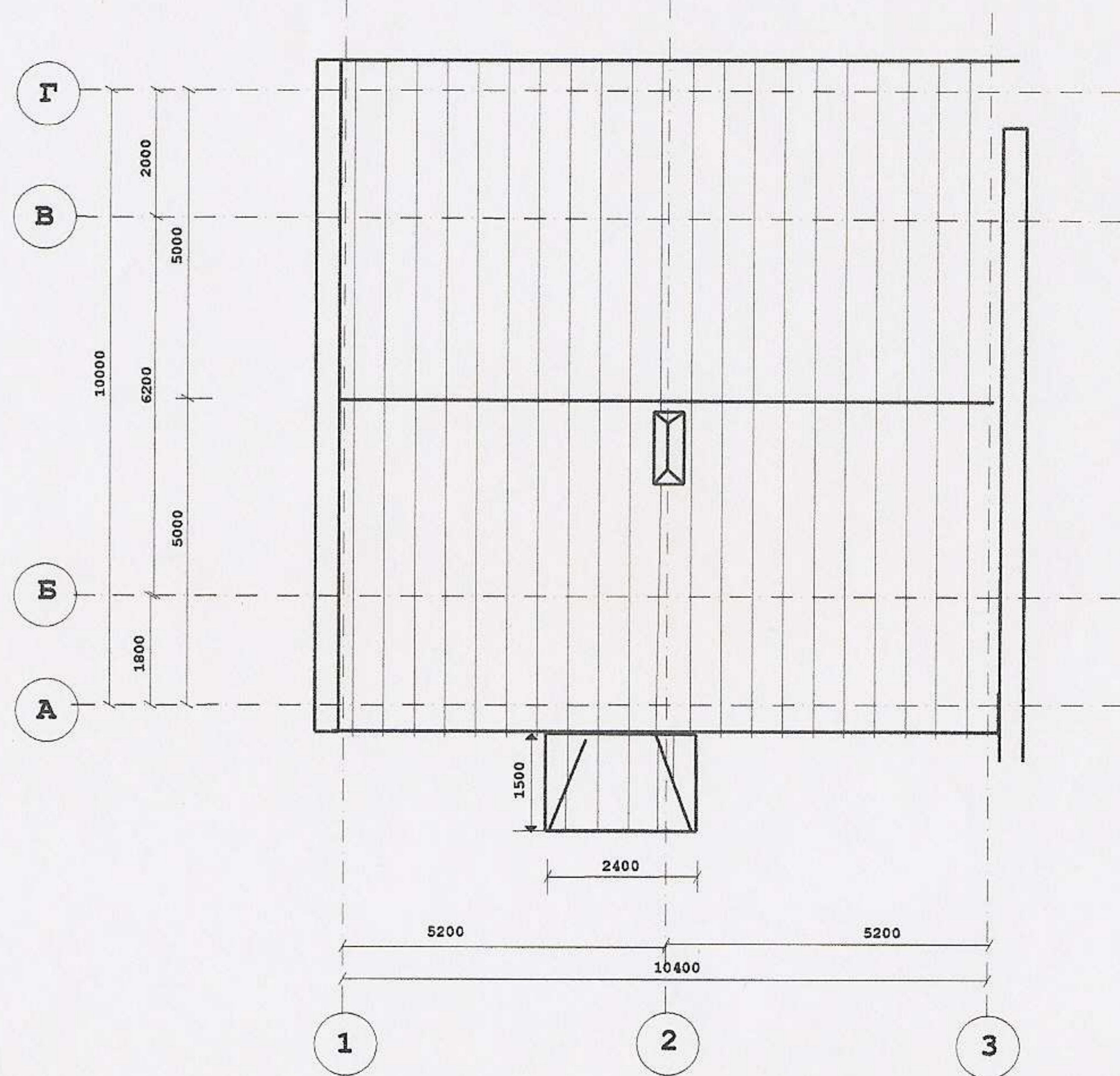
План кровли
