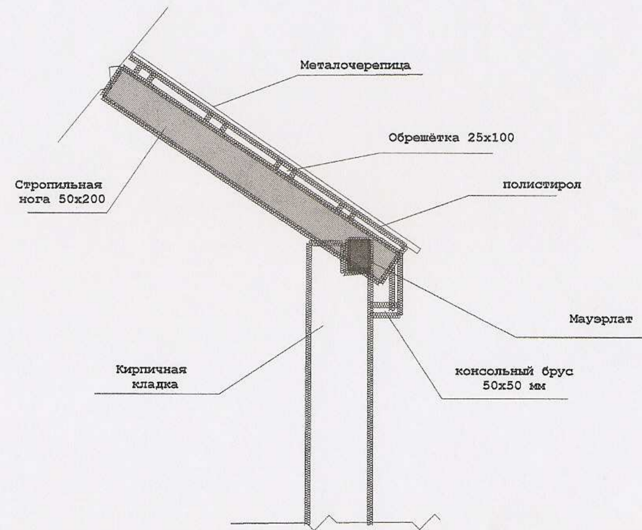
Разрез карниза
