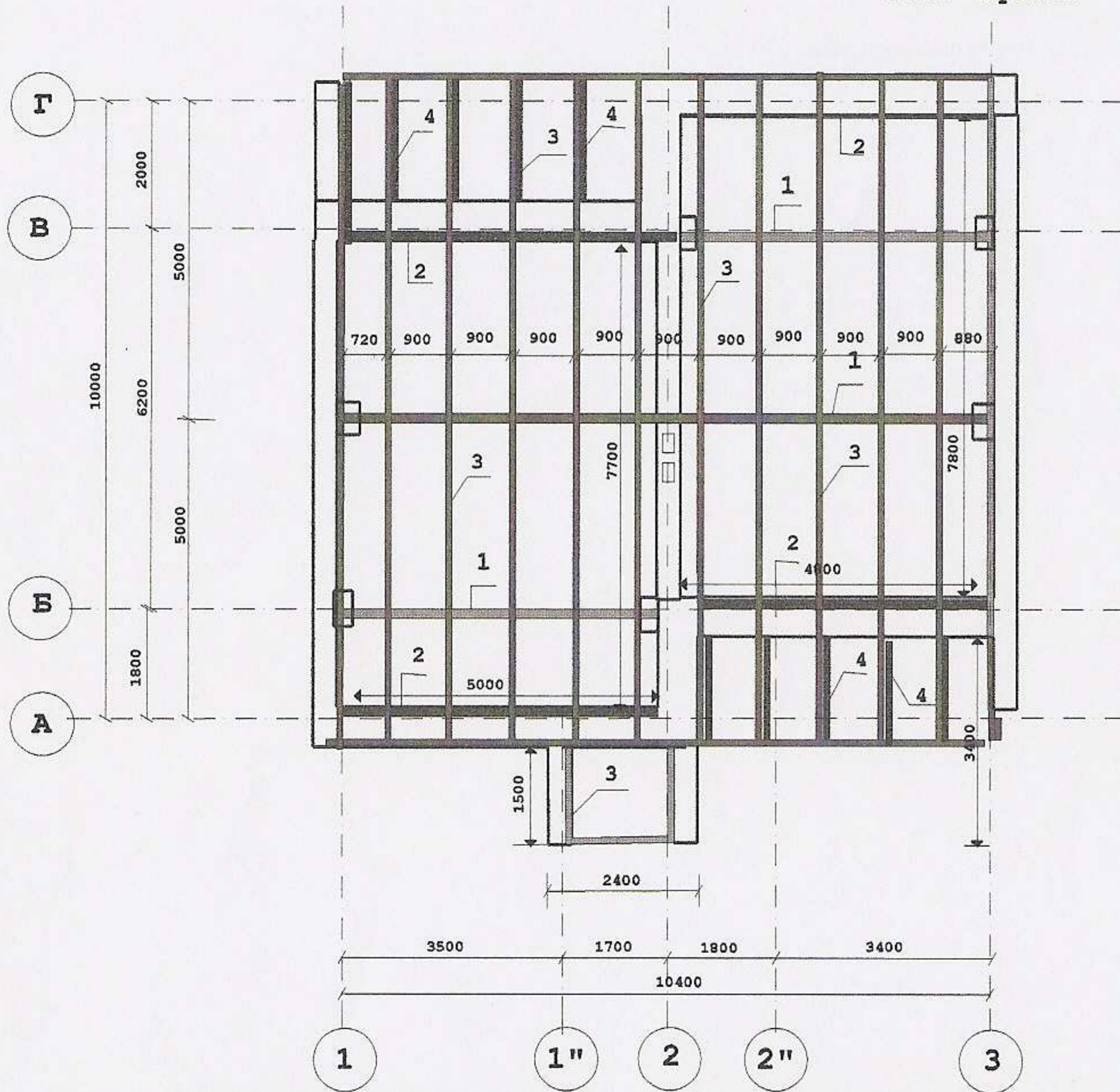
План стропил
